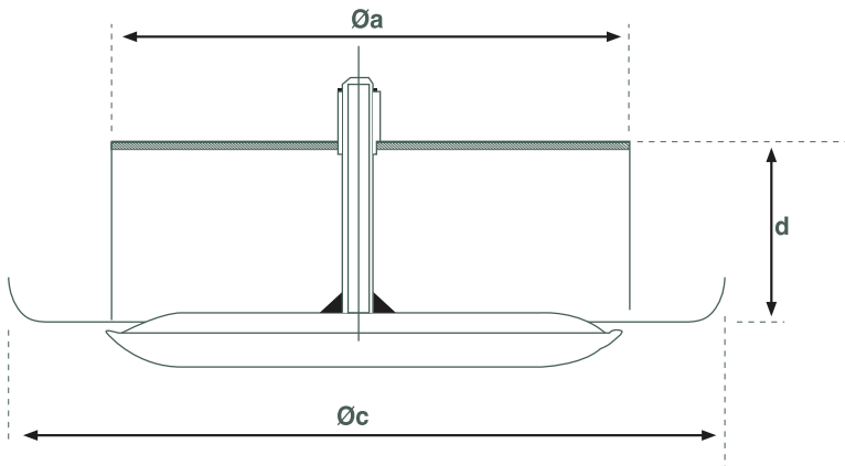
Gemici Anemostadı Kesidi Disc Valve Section
